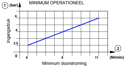
KARAKTERISTIEK DOORSTROMING MINIMUM OPERATIONEEL
