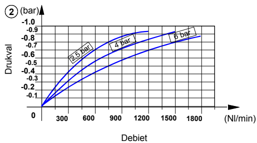
KARAKTERISTIEK DOORSTROMING
